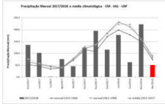
Figura 1: Precipitação mensal de maio de 2017 a abril de 2018, além de médias e normais climatológicas.
