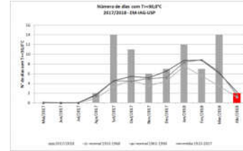
Figura 3: Número de dias com T>=30,0°C de maio de 2017 a abril de 2018, além de médias e normais climatológicas.
