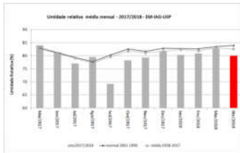
Figura 7: Umidade relativa média mensal de maio de 2017 a abril de 2018, além de médias e normais climatológicas.
