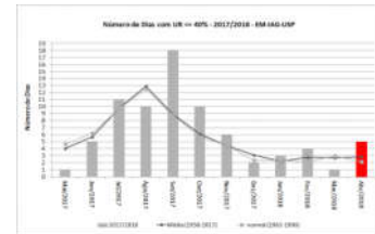
Figura 9: Número mensal de dias com UR<=40% de maio de 2017 a abril de 2018, além de médias e normais climatológicas.
