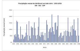
Figura 2: Precipitação mensal em abril de 1933 a 2018.
