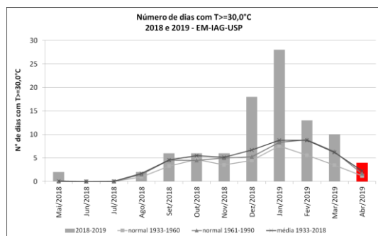
Figura 3: Número de dias com T≥30,0°C de maio de 2018 a abril de 2019, além de médias e normais climatológicas.
