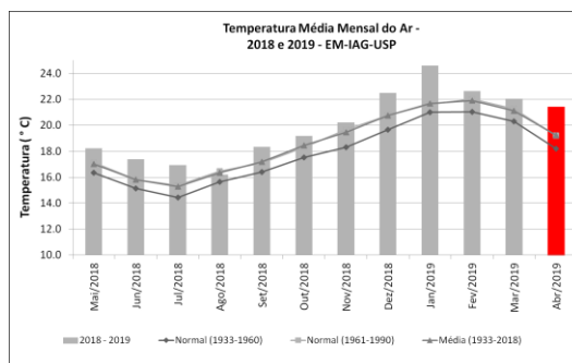
Figura 4: Temperatura média mensal de maio de 2018 a abril de 2019, além de médias e normais climatológicas.
