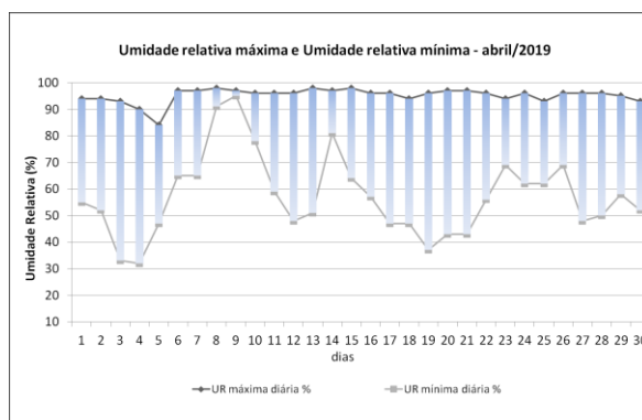
Figura 11 – Umidade relativa máxima diária e umidade relativa mínima diária em abril de 2019. As barras representam a amplitude diária.
