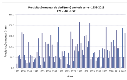
Figura 2: Precipitação mensal acumulada em abril de 1933 a 2019.
