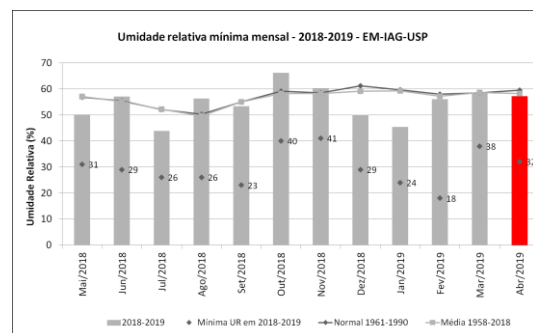
Figura 8: Umidade relativa média mínima mensal e mínimas mensais de maio de 2018 a abril de 2019, além de médias e normais climatológicas.
