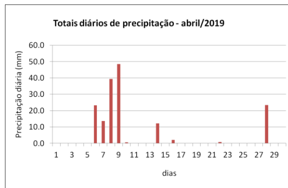
Figura 12 – Totais diários de precipitação registrados em abril de 2019.
