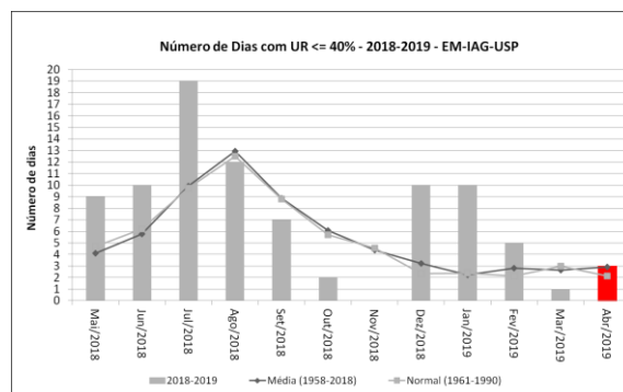
Figura 9: Número mensal de dias com UR<=40% de maio de 2018 a abril de 2019, além de médias e normais climatológicas.
