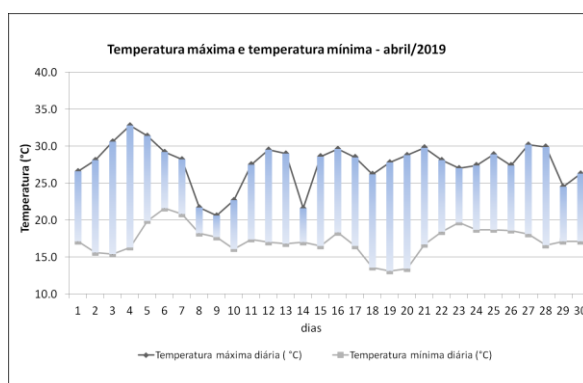
Figura 10 - Temperatura máxima diária e temperatura mínima diária para abril de 2019. As barras representam a amplitude diária.
