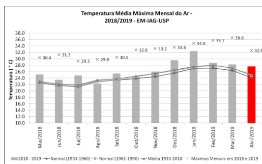
Figura 5: Valores médios mensais de temperatura máxima e valor máximo registrado da temperatura do ar em cada mês, de maio de 2018 a abril de 2019, além de médias e normais climatológicas.
