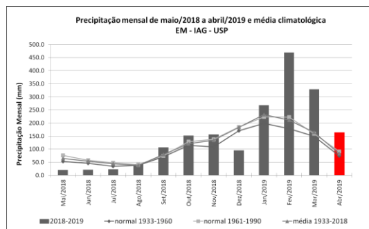
Figura 1: Precipitação acumulada mensal de maio de 2018 a abril de 2019, além de médias e normais climatológicas.
