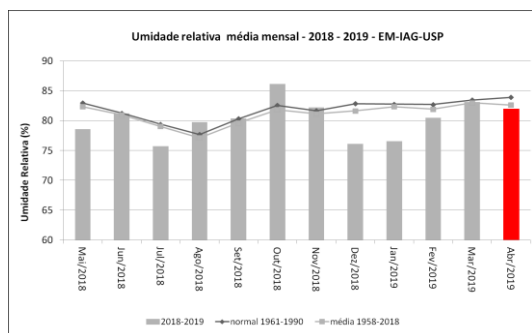
Figura 7: Umidade relativa média mensal de maio de 2018 a abril de 2019, além de médias e normais climatológicas.
