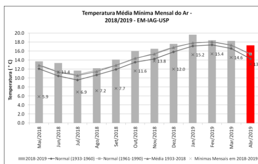
Figura 6: Valores médios mensais de temperatura mínima e valor mínimo registrado da temperatura do ar em cada mês, de maio de 2018 a abril de 2019, além de médias e normais climatológicas.
