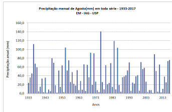
Figura 2: Precipitação mensal em agosto de 1933 a 2017.
