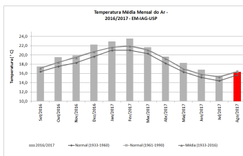
Figura 4: Temperatura média de setembro de 2016 a agosto de 2017, além de médias e normais climatológicas.
