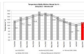
Figura 6: Valores médios mensais de temperatura mínima e valor mínimo registrado da temperatura do ar em cada mês, de setembro de 2016 a agosto de 2017, além de médias e normais climatológicas.
