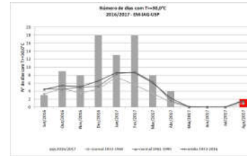
Figura 3: Número de dias com T>=30,0°C de setembro de 2016 a agosto de 2017, além de médias e normais climatológicas.
