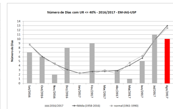
Figura 9: Número mensal de dias com UR<=40% de setembro de 2016 a agosto de 2017, além de médias e normais climatológicas.
