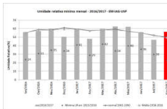
Figura 8: Médias mensais da umidade relativa mínima e valores mínimos mensais de umidade relativa de setembro de 2016 a agosto de 2017, além de médias e normais climatológicas.
