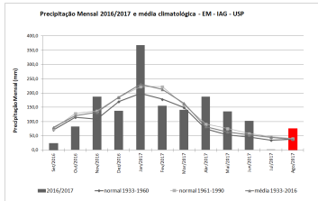
Figura 1: Precipitação mensal de setembro de 2016 a agosto de 2017, além de médias e normais climatológicas.
