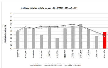
Figura 7: Umidade relativa média mensal de setembro de 2016 a agosto de 2017, além de médias e normais climatológicas.
