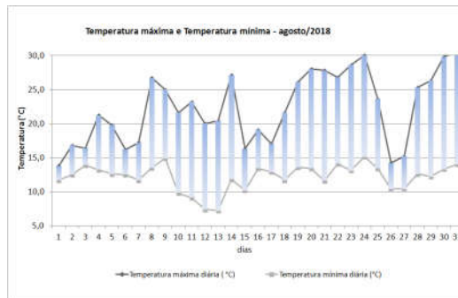
Figura 10 - Temperatura máxima diária e temperatura mínima diária. As barras representam a amplitude diária. Mês de agosto/2018
