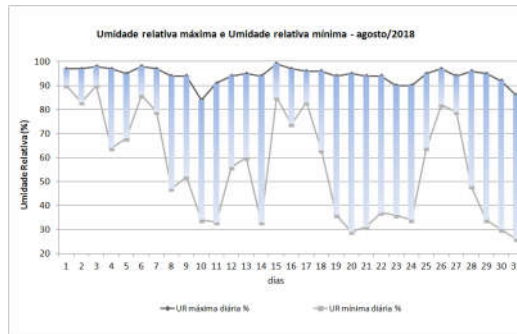
Figura 11 – Umidade relativa máxima diária e umidade relativa mínima diária. As barras representam a amplitude diária. Mês de agosto/2018
