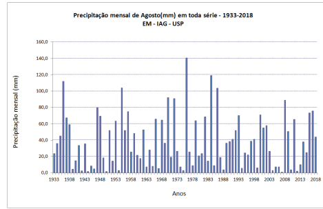
Figura 2: Precipitação mensal acumulada em agosto de 1933 a 2018.
