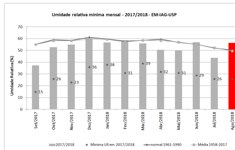
Figura 8: Umidade relativa média mínima mensal e mínimos mensais de setembro de 2017 a agosto de 2018, além de médias e normais climatológicas.
