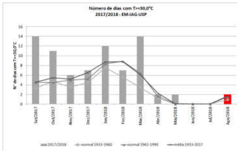
Figura 3: Número de dias com T>=30,0°C de setembro de 2017 a agosto de 2018, além de médias e normais climatológicas.
