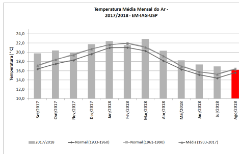
Figura 4: Temperatura média mensal de setembro de 2017 a agosto de 2018, além de médias e normais climatológicas.
