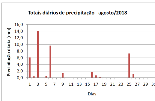
Figura 12 – Totais diários de precipitação – agosto/2018
