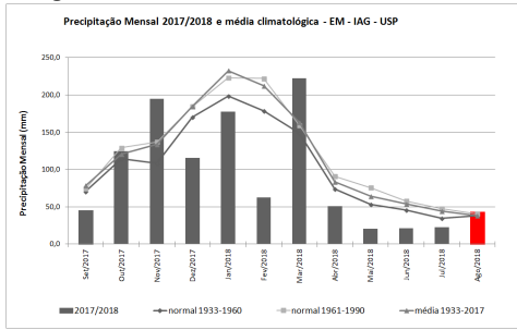
Figura 1: Precipitação acumulada mensal de setembro de 2017 a agosto de 2018, além de médias e normais climatológicas.
