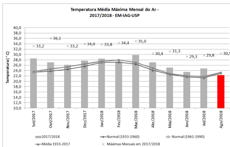
Figura 5: Valores médios mensais de temperatura máxima e valor máximo registrado da temperatura do ar em cada mês, de setembro de 2017 a agosto de 2018, além de médias e normais climatológicas.
