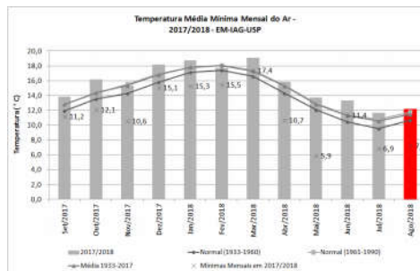
Figura 6: Valores médios mensais de temperatura mínima e valor mínimo registrado da temperatura do ar em cada mês, de setembro de 2017 a agosto de 2018, além de médias e normais climatológicas.
