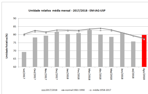
Figura 7: Umidade relativa média mensal de setembro de 2017 a agosto de 2018, além de médias e normais climatológicas.
