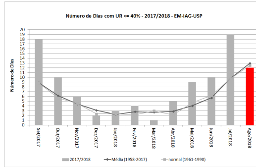
Figura 9: Número mensal de dias com UR<=40% de setembro de 2017 a agosto de 2018, além de médias e normais climatológicas.
