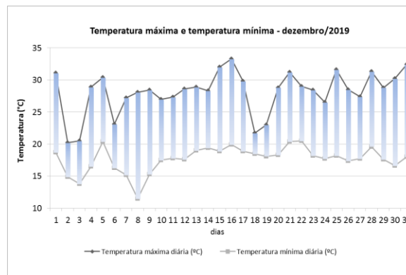
Figura 10 - Temperatura máxima diária e temperatura mínima diária para dezembro de 2019. As barras representam a amplitude diária.
