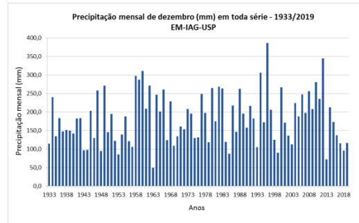
Figura 2: Precipitação mensal acumulada em dezembro de 1933 a 2019.
