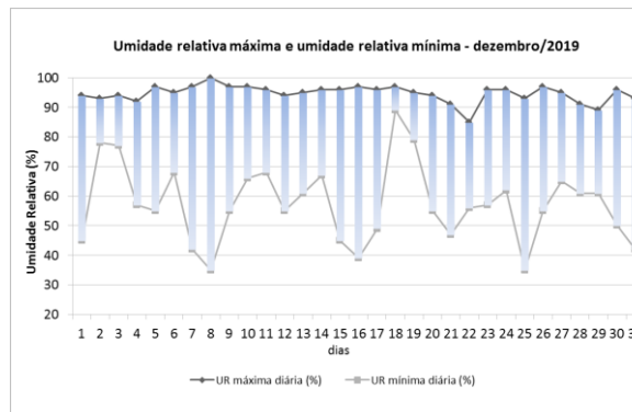
Figura 11 – Umidade relativa máxima diária e umidade relativa mínima diária em dezembro de 2019. As barras representam a amplitude diária.
