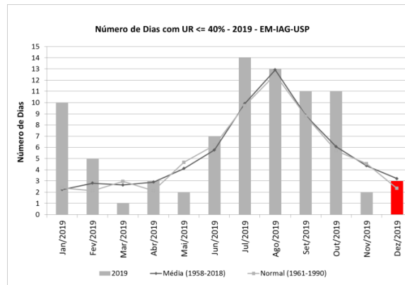
Figura 9: Número mensal de dias com UR<=40% de janeiro de 2019 a dezembro de 2019, além de médias e normais climatológicas.
