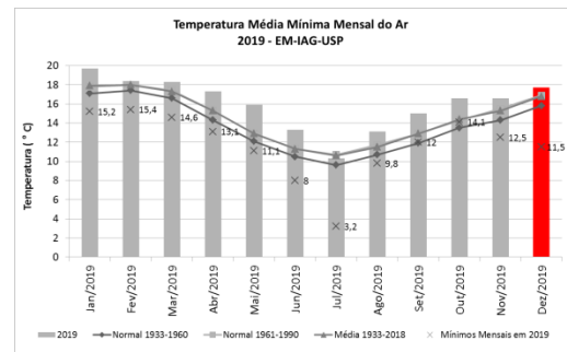
Figura 6: Valores médios mensais de temperatura mínima e valor mínimo registrado da temperatura do ar em cada mês, de janeiro de 2019 a dezembro de 2019, além de médias e normais climatológicas.
