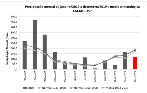
Figura 1: Precipitação acumulada mensal de janeiro de 2019 a dezembro de 2019, além de médias e normais climatológicas.
