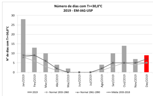
Figura 3: Número de dias com T \geq 30,0^\circ\text{C} de janeiro de 2019 a dezembro de 2019, além de médias e normais climatológicas.
