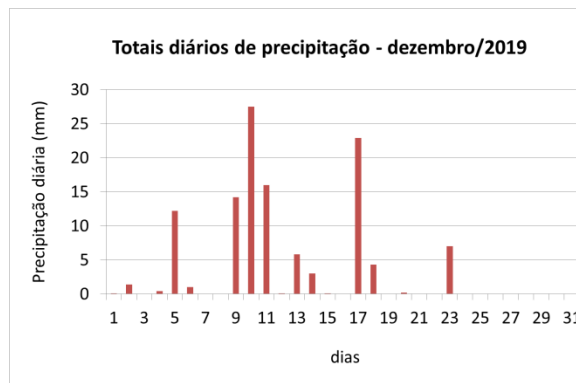
Figura 12 – Totais diários de precipitação registrados em dezembro de 2019.
