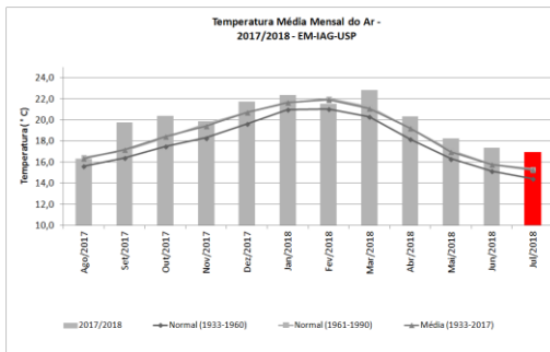
Figura 4: Temperatura média mensal de agosto de 2017 a julho de 2018, além de médias e normais climatológicas.
