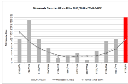
Figura 9: Número mensal de dias com UR<=40% de agosto de 2017 a julho de 2018, além de médias e normais climatológicas.
