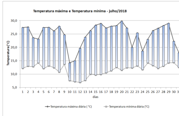
Figura 10 - Temperatura máxima diária e temperatura mínima diária. As barras representam a amplitude diária. Mês de julho/2018
