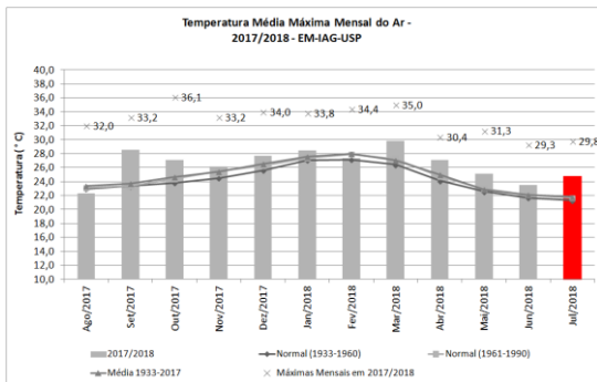
Figura 5: Valores médios mensais de temperatura máxima e valor máximo registrado da temperatura do ar em cada mês, de agosto de 2017 a julho de 2018, além de médias e normais climatológicas.
