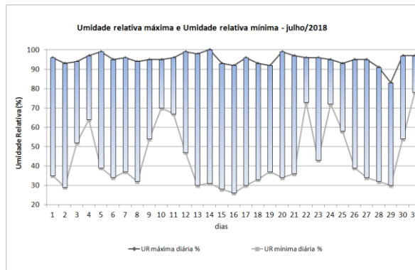
Figura 11 – Umidade relativa máxima diária e umidade relativa mínima diária. As barras representam a amplitude diária. Mês de julho/2018
