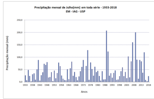
Figura 2: Precipitação mensal acumulada em julho de 1933 a 2018.
