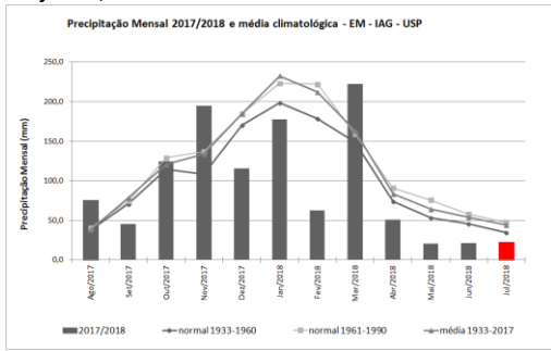
Figura 1: Precipitação acumulada mensal de agosto de 2017 a julho de 2018, além de médias e normais climatológicas.
