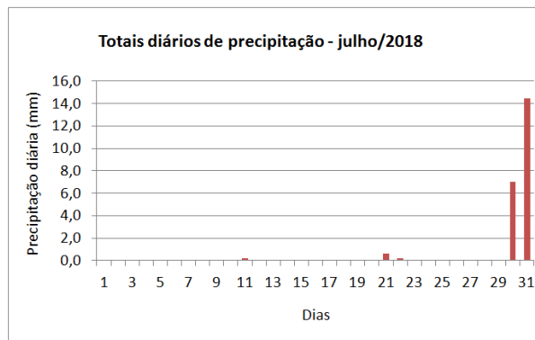
Figura 12 – Totais diários de precipitação – julho/2018
