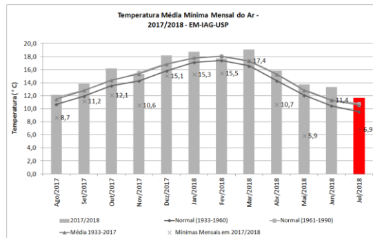
Figura 6: Valores médios mensais de temperatura mínima e valor mínimo registrado da temperatura do ar em cada mês, de agosto de 2017 a julho de 2018, além de médias e normais climatológicas.
