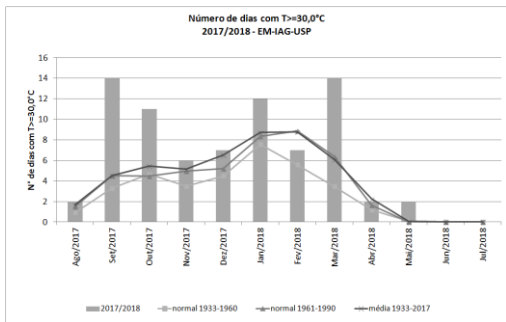
Figura 3: Número de dias com T>=30,0°C de agosto de 2017 a julho de 2018, além de médias e normais climatológicas.
