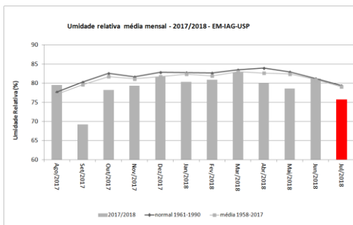
Figura 7: Umidade relativa média mensal de agosto de 2017 a julho de 2018, além de médias e normais climatológicas.
