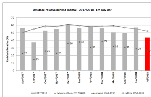
Figura 8: Umidade relativa média mínima mensal e mínimas mensais de agosto de 2017 a julho de 2018, além de médias e normais climatológicas.
