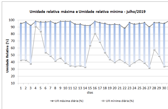
Figura 11 – Umidade relativa máxima diária e umidade relativa mínima diária em julho de 2019. As barras representam a amplitude diária.
