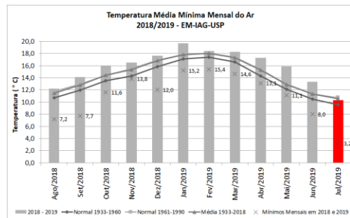
Figura 6: Valores médios mensais de temperatura mínima e valor mínimo registrado da temperatura do ar em cada mês, de agosto de 2018 a julho de 2019, além de médias e normais climatológicas.
