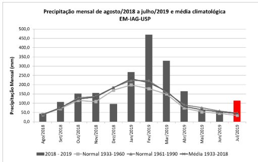
Figura 1: Precipitação acumulada mensal de agosto de 2018 a julho de 2019, além de médias e normais climatológicas.
