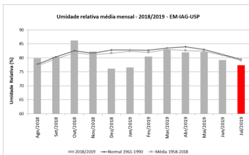
Figura 7: Umidade relativa média mensal de agosto de 2018 a julho de 2019, além de médias e normais climatológicas.
