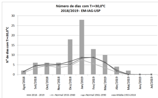
Figura 3: Número de dias com T>=30,0°C de agosto de 2018 a julho de 2019, além de médias e normais climatológicas.
