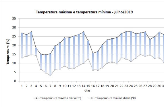
Figura 10 - Temperatura máxima diária e temperatura mínima diária para julho de 2019. As barras representam a amplitude diária.
