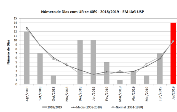
Figura 9: Número mensal de dias com UR≤40% de agosto de 2018 a julho de 2019, além de médias e normais climatológicas.
