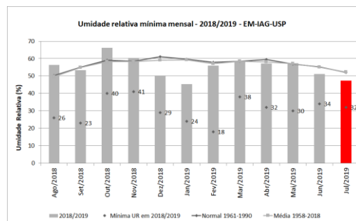
Figura 8: Umidade relativa média mínima mensal e mínimas mensais de agosto de 2018 a julho de 2019, além de médias e normais climatológicas.
