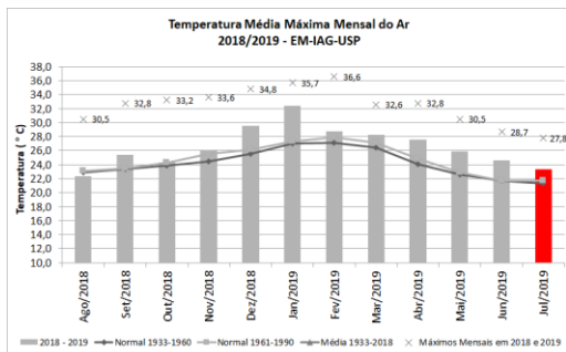
Figura 5: Valores médios mensais de temperatura máxima e valor máximo registrado da temperatura do ar em cada mês, de agosto de 2018 a julho de 2019, além de médias e normais climatológicas.
