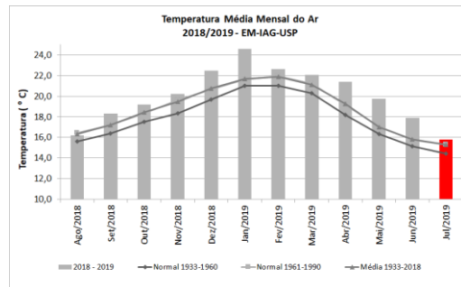
Figura 4: Temperatura média mensal de agosto de 2018 a julho de 2019, além de médias e normais climatológicas.
