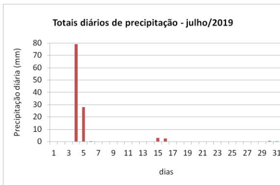
Figura 12 – Totais diários de precipitação registrados em julho de 2019.
