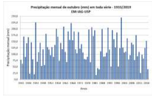
Figura 2: Precipitação mensal acumulada em outubro de 1933 a 2019.
