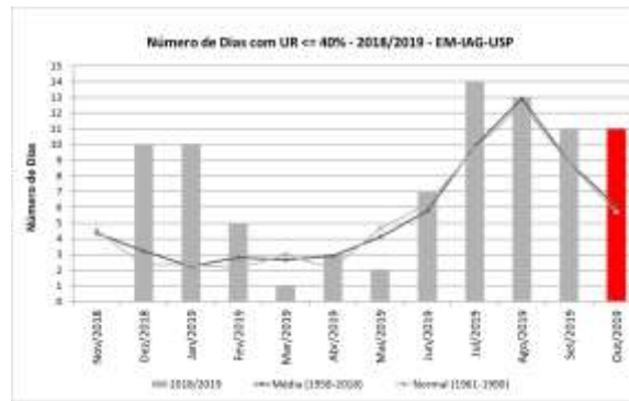
Figura 9: Número mensal de dias com UR<=40% de novembro de 2018 a outubro de 2019, além de médias e normais climatológicas.
