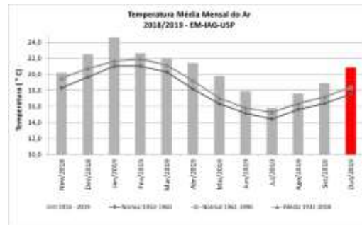
Figura 4: Temperatura média mensal de novembro de 2018 a outubro de 2019, além de médias e normais climatológicas.
