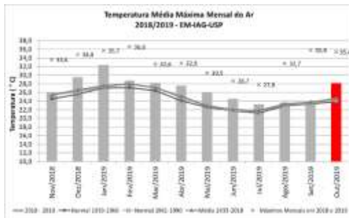
Figura 5: Valores médios mensais de temperatura máxima e valor máximo registrado da temperatura do ar em cada mês, de novembro de 2018 a outubro de 2019, além de médias e normais climatológicas.
