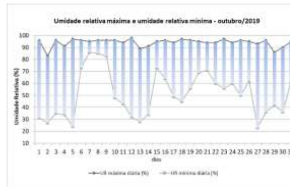
Figura 11 – Umidade relativa máxima diária e umidade relativa mínima diária em outubro de 2019. As barras representam a amplitude diária.
