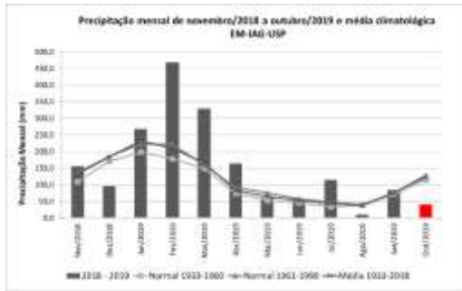
Figura 1: Precipitação acumulada mensal de novembro de 2018 a outubro de 2019, além de médias e normais climatológicas.
