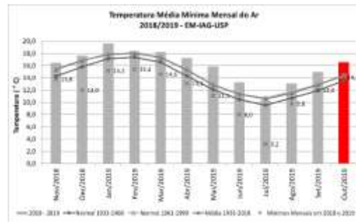
Figura 6: Valores médios mensais de temperatura mínima e valor mínimo registrado da temperatura do ar em cada mês, de novembro de 2018 a outubro de 2019, além de médias e normais climatológicas.
