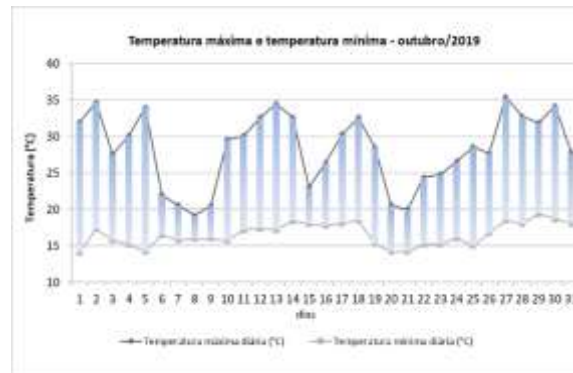
Figura 10 - Temperatura máxima diária e temperatura mínima diária para outubro de 2019. As barras representam a amplitude diária.
