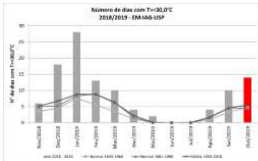
Figura 3: Número de dias com T \geq 30,0^{\circ}\text{C} de novembro de 2018 a outubro de 2019, além de médias e normais climatológicas.
