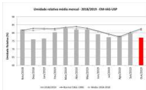
Figura 7: Umidade relativa média mensal de novembro de 2018 a outubro de 2019, além de médias e normais climatológicas.
