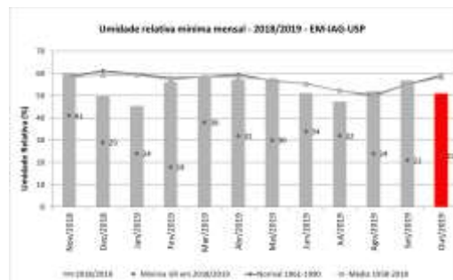
Figura 8: Umidade relativa média mínima mensal e mínimas mensais de novembro de 2018 a outubro de 2019, além de médias e normais climatológicas.
