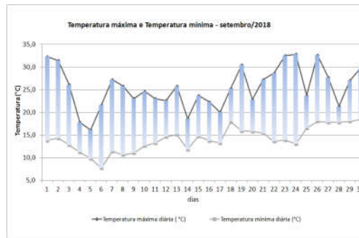
Figura 10 - Temperatura máxima diária e temperatura mínima diária. As barras representam a amplitude diária. Mês de setembro/2018
