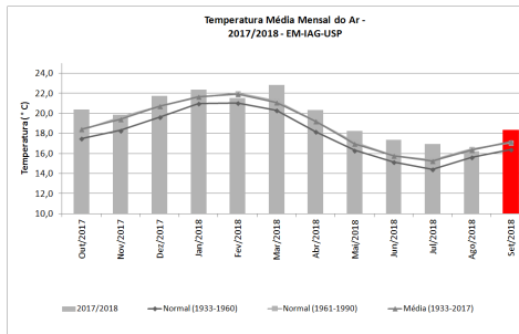
Figura 4: Temperatura média mensal de outubro de 2017 a setembro de 2018, além de médias e normais climatológicas.
