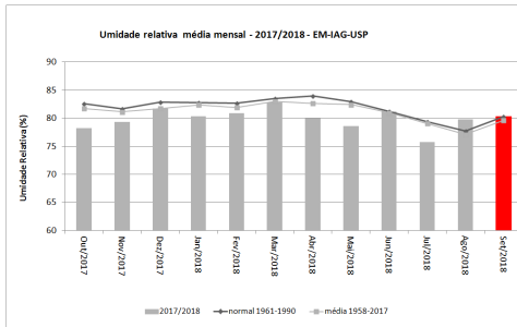
Figura 7: Umidade relativa média mensal de outubro de 2017 a setembro de 2018, além de médias e normais climatológicas.
