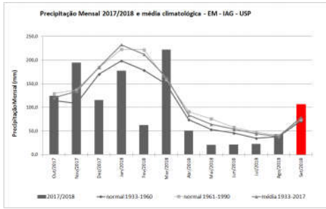
Figura 1: Precipitação acumulada mensal de outubro de 2017 a setembro de 2018, além de médias e normais climatológicas.
