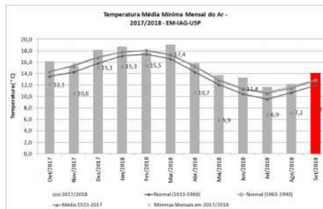
Figura 6: Valores médios mensais de temperatura mínima e valor mínimo registrado da temperatura do ar em cada mês, de outubro de 2017 a setembro de 2018, além de médias e normais climatológicas.
