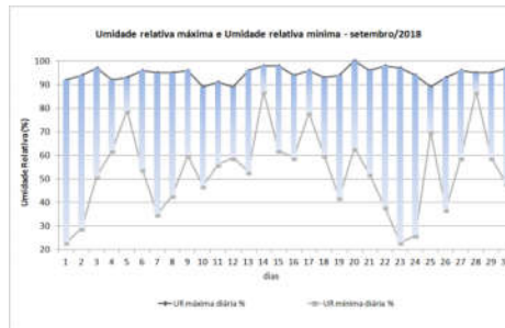
Figura 11 – Umidade relativa máxima diária e umidade relativa mínima diária. As barras representam a amplitude diária. Mês de setembro/2018
