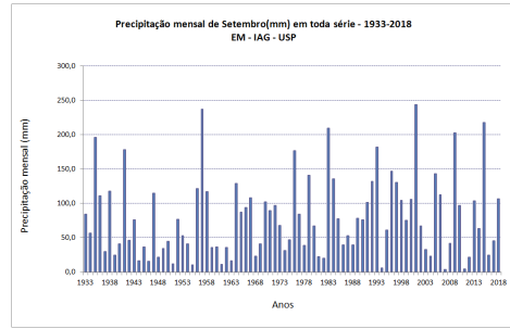
Figura 2: Precipitação mensal acumulada em setembro de 1933 a 2018.
