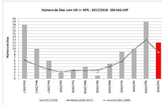
Figura 9: Número mensal de dias com UR<=40% de outubro de 2017 a setembro de 2018, além de médias e normais climatológicas.
