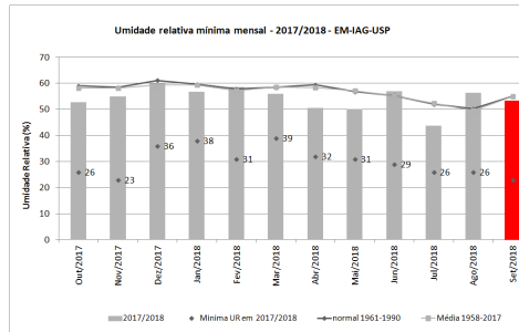
Figura 8: Umidade relativa média mínima mensal e mínimas mensais de outubro de 2017 a setembro de 2018, além de médias e normais climatológicas.
