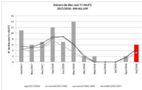
Figura 3: Número de dias com T>=30,0°C de outubro de 2017 a setembro de 2018, além de médias e normais climatológicas.
