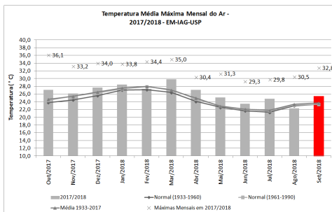
Figura 5: Valores médios mensais de temperatura máxima e valor máximo registrado da temperatura do ar em cada mês, de outubro de 2017 a setembro de 2018, além de médias e normais climatológicas.
