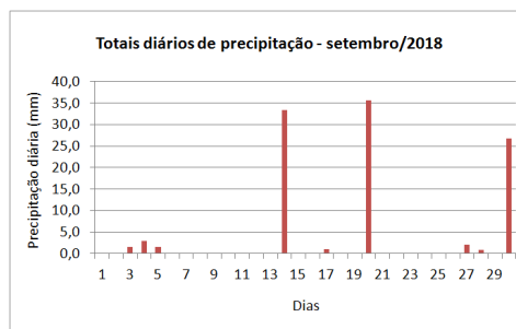
Figura 12 – Totais diários de precipitação – setembro/2018
